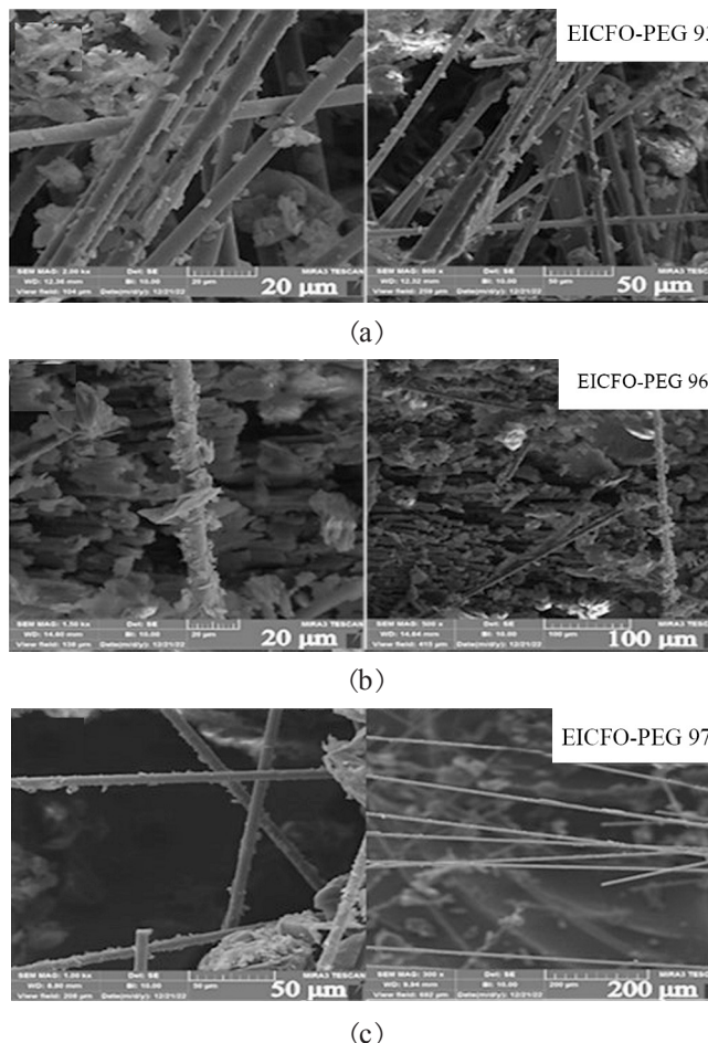
شکل ۶- تصاویر FE-SEM از نمونه های کامپوزیتی تغییر فاز (a) EICFO-PEG93 با بزرگنمایی ۲۰ و ۵۰ μm (b) EICFO-PEG96 با بزرگنمایی ۲۰ و ۱۰۰ μm و (c) EICFO-PEG97 با بزرگنمایی ۲۰۰ و ۵۰ μm.
