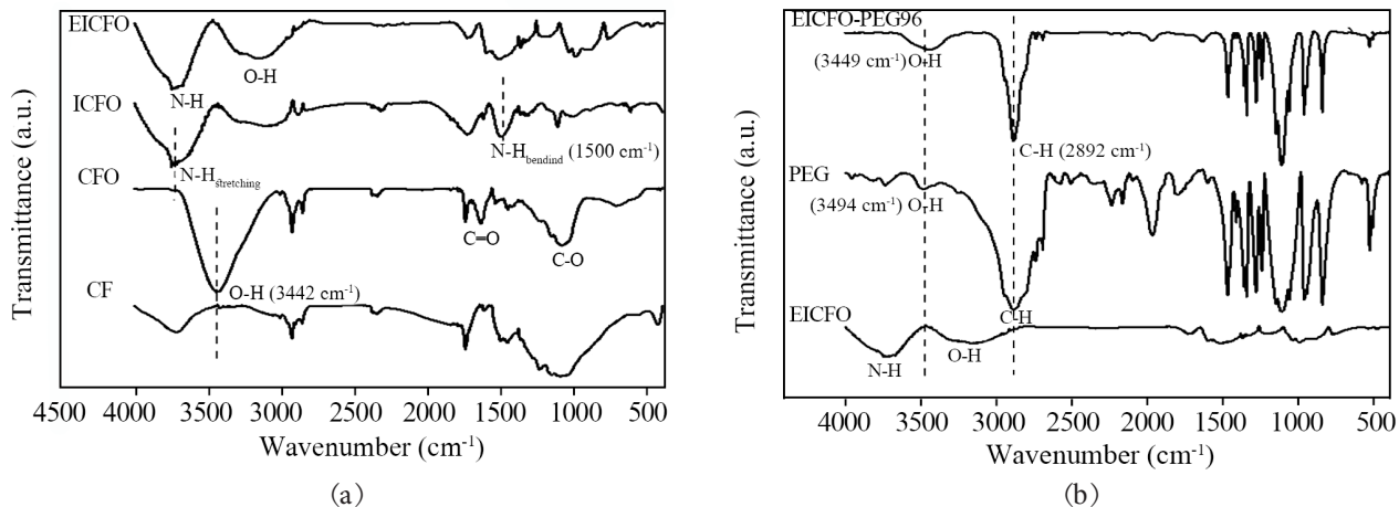
شکل ۲- طیف‌های FTIR: (a) تکرار شده کربن خالص و اصلاح شده و (b) پلی (اتیلن گلیکول) و نمونه کامپوزیتی تغییر فاز مطلوب (EICFO-PEG-96). Fig. 2. FTIR spectra of: (a) pure and modified carbon monofilament and (b) poly(ethylene glycol) and desired phase change composite sample (EICFO-PEG-96).
