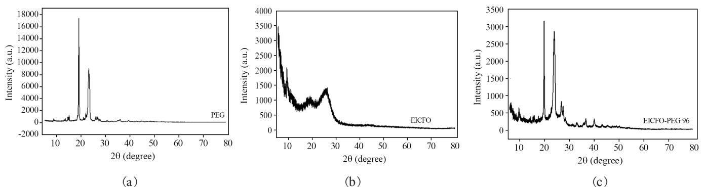
شکل ۴- الگوهای XRD: (a) پلی (اتیلن گلیکول) خالص، (b) تکرشته کربن اصلاح شده (EICFO) و (c) نمونه مطلوب (EICFO-PEG 96). Fig. 4. XRD patterns of: (a) pure polyethylene glycol (PEG), (b) modified carbon monofilament (EICFO), and (c) desired sample (EICFO-PEG 96).
