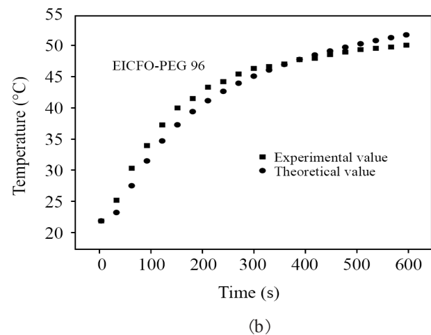
شکل ۹- مقایسه منحنی تجربی و نظری دما برحسب زمان برای (a) نمونه شاهد (CS) و (b) نمونه مطلوب (EICFO-PEG 96). Fig. 9. Comparison of the experimental and theoretical temperature curves versus time for (a) the control sample (CS) and (b) the desired sample (EICFO-PEG 96).
